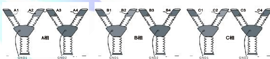
十二断口信号线的连接
