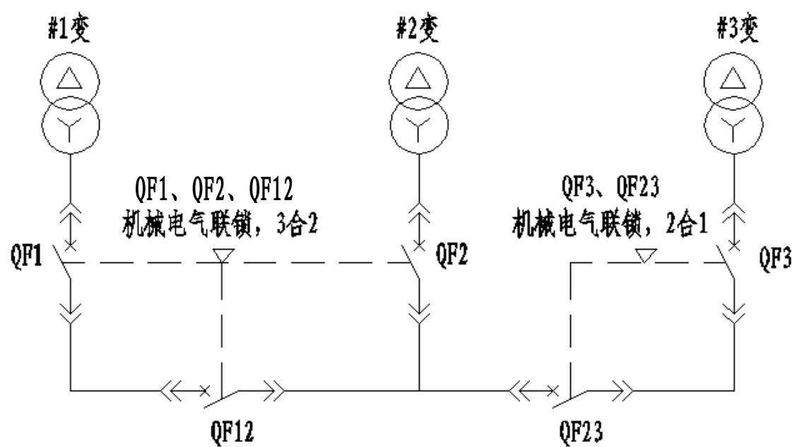
3台变压器低压联锁示意图
