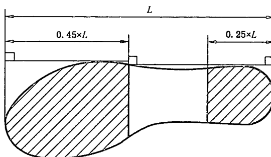
图 2 防滑花纹
